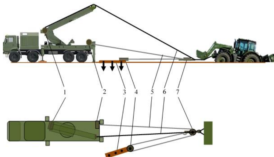
Рисунок 1 – Комбинированный способ вытаскивания
