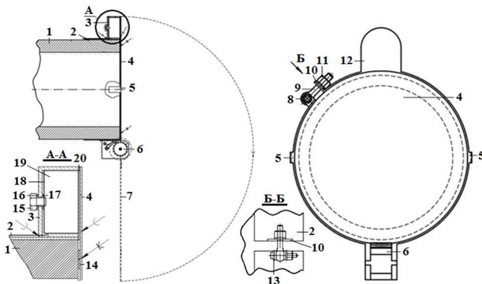
Рис.1. Уплотнение дульного среза пушки:
