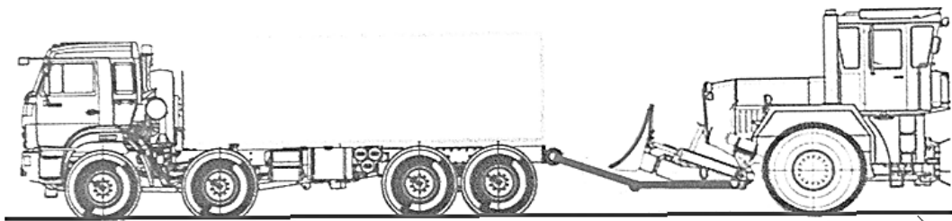
Рисунок 3 – Схема жесткой сцепки РЭМ и ИТ с бульдозерным оборудованием
