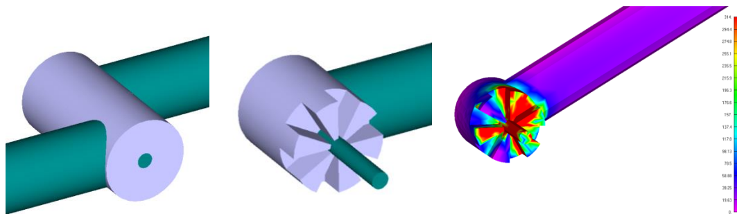
Рисунок 5 – Механизм излома штанг буксира в виде фланцев с пальцами
