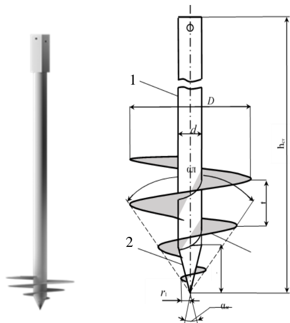
Рисунок 2 Грунтовой винтовой анкер где: 1 – ствол; 2- конусный наконечник; 3 – винтовая лопасть
