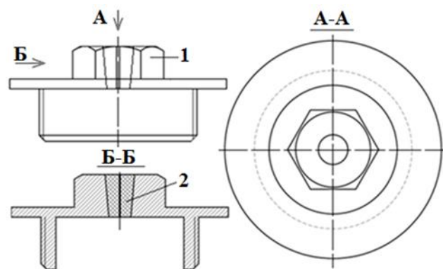
Рис. 3. Крышка корпуса коробки 4Т: 1 – крышка; 2 – конусный резиновый уплотнитель ГОСТ 53820-2010
