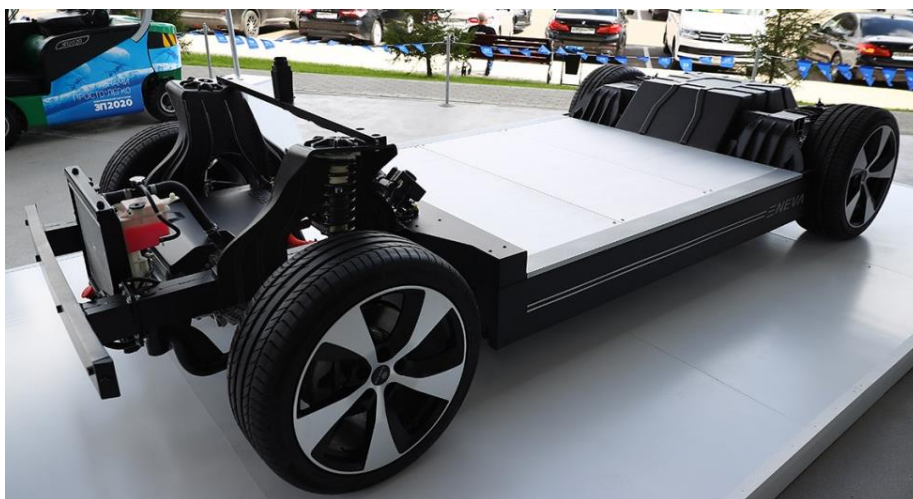
Рис 1. Беспилотная модульная электрическая платформа.
