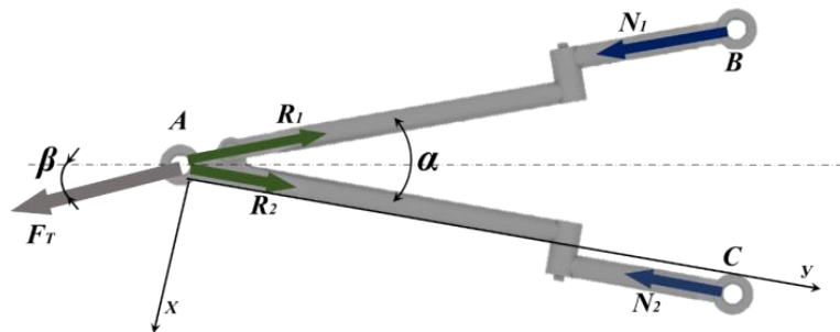
Рисунок 4– Расчетная схема нагружения буксира при движении автопоезда вперед с поворотом налево
